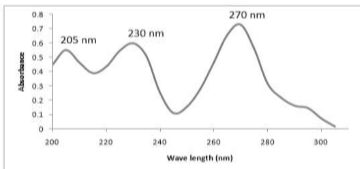
Fig. 11. Absorption spectrum of ferrioin ( 1 \times 10^{-5} M).
